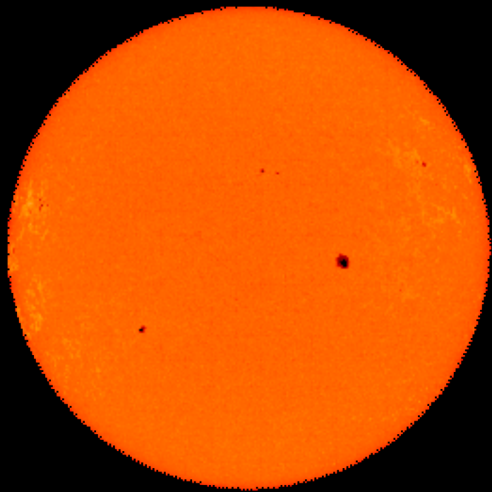
Sun
