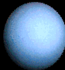
Uranus
