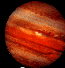
Jupiter
